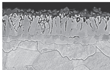
断面 SEM 像
